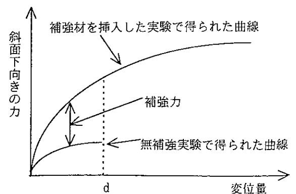
図-1 補強力の概念図
