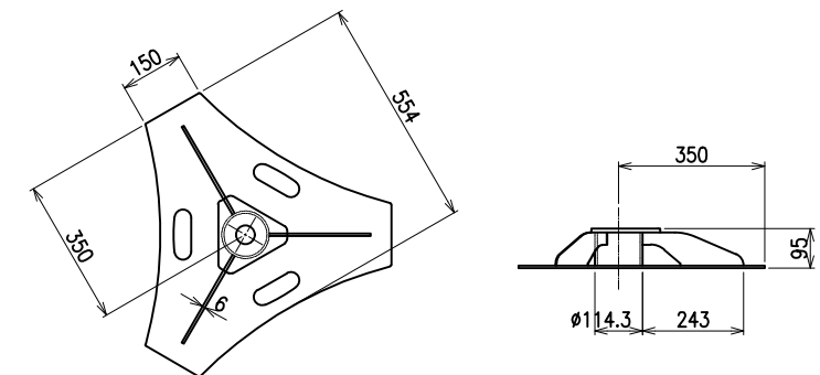
支圧板 S=1/10
