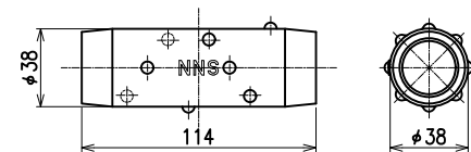
ファイアローブ・ターンバックル S=1/3
