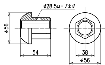
NNS突起付カプラ S=1/2
