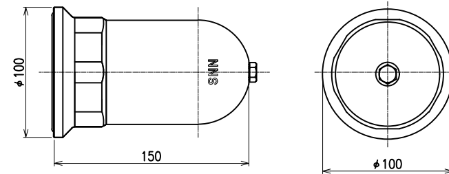
NNS蛇腹シーブ S=1/3
