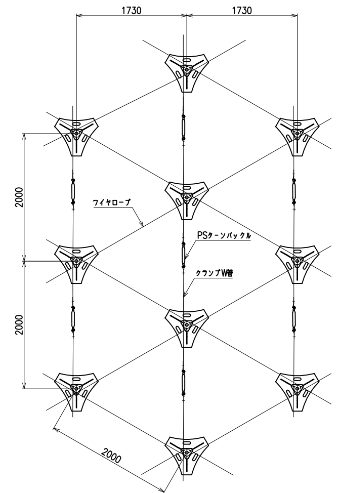
配置例 S=1/30
