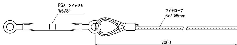
ファイアローブ・ターンバックル S=1/3
