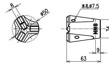
NNSビット S=1/2
