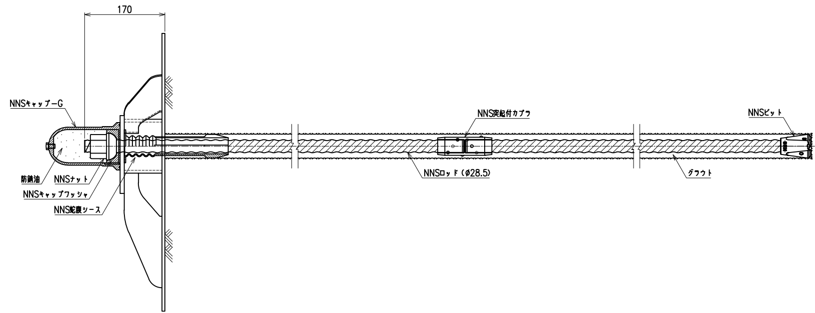
構造概要図 S=1/4
